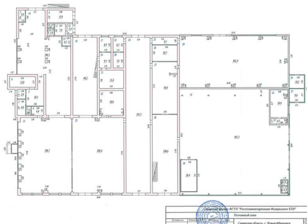
План 1 этажа лит.А,А1,А2,а
