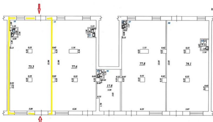
План 1 этажа лит. С
